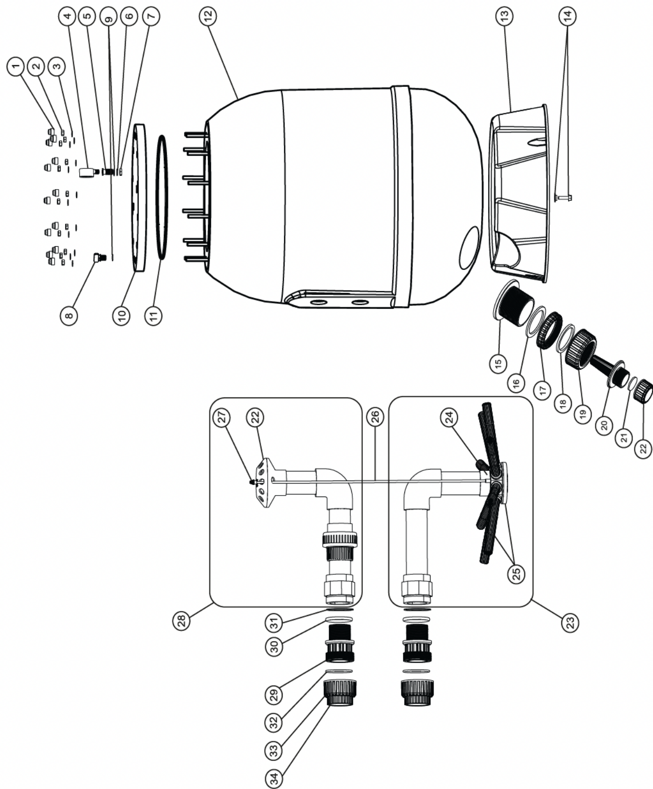
SCHÉMA ÉCLATÉ
