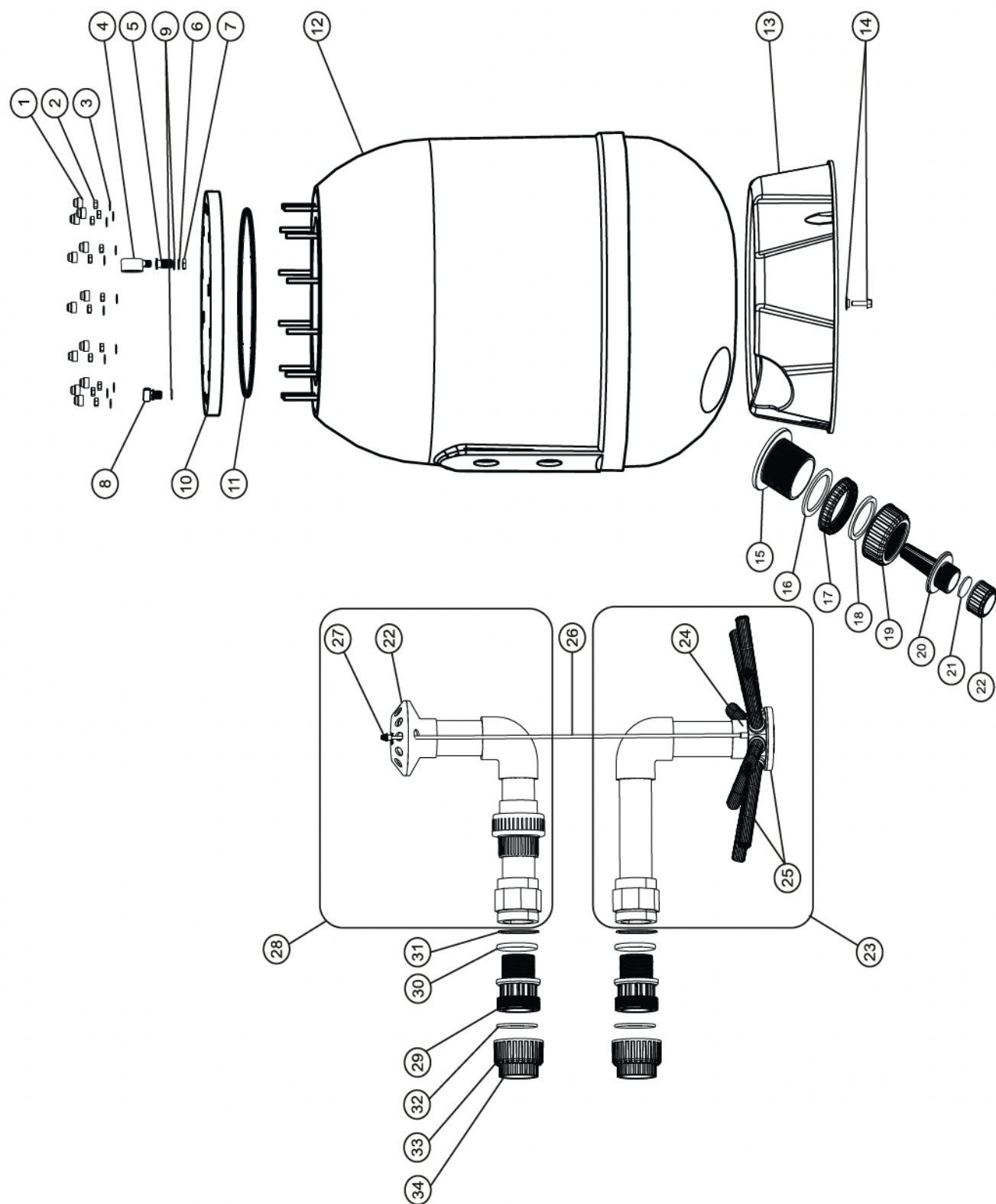
UPPDELAD DIAGRAM
